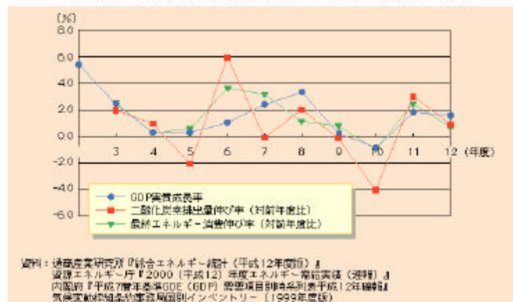
図2-3-3 GDP成長率、CO 2 排出量伸び率、エネルギー消費伸び率の関係
