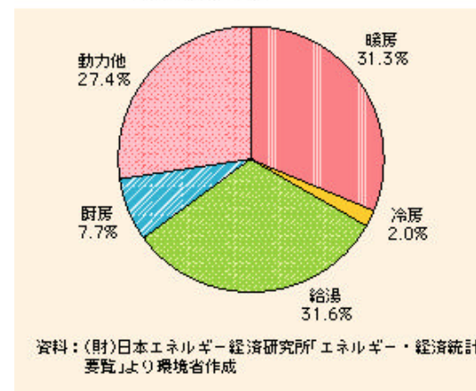
図3-4-3 民生家庭部門における二酸化炭素排出量の 内訳(2005年度)
